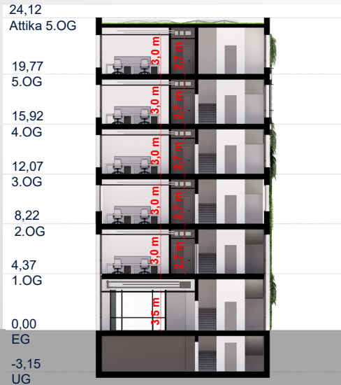
Schnitt A-A
